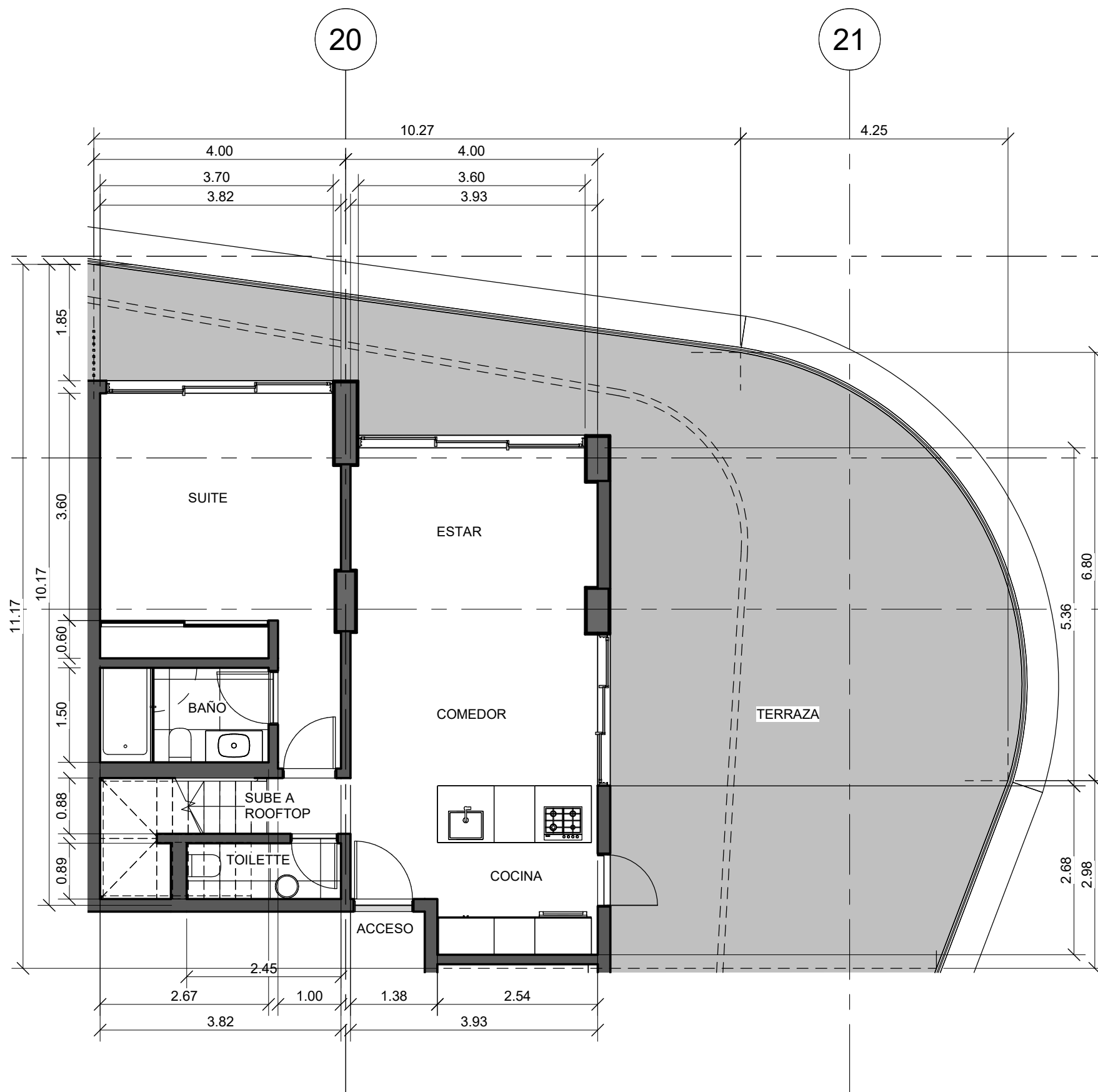
1-UF 83 PB 1 : 75
