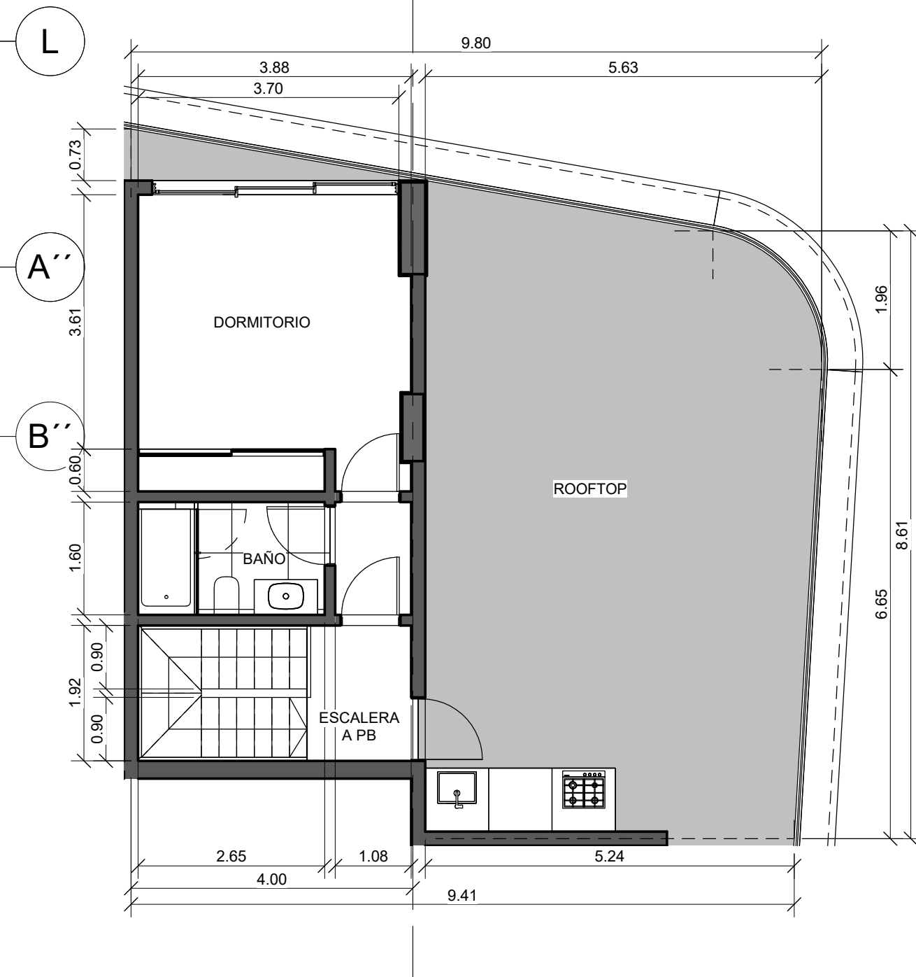
2-UF 83 ROOFTOP 1 : 75
