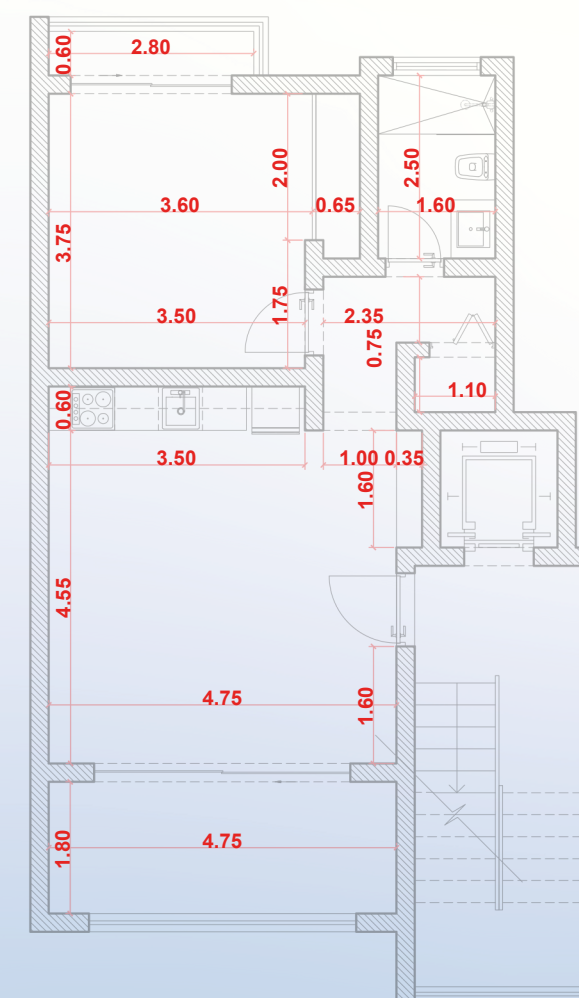
PLANTA DIMENSIONADA
