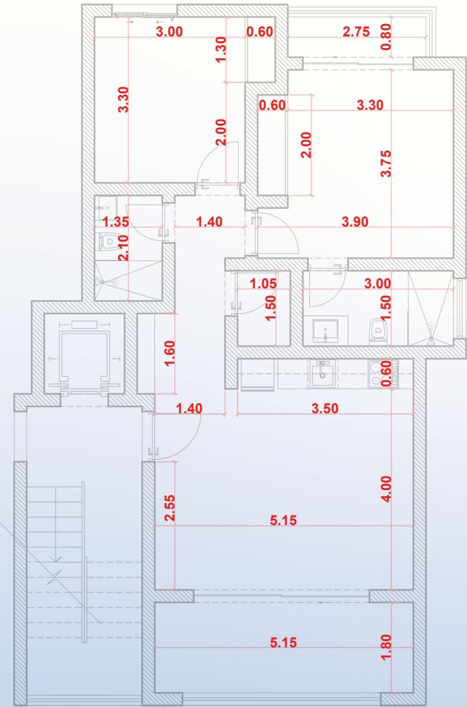
PLANTA DIMENSIONADA
