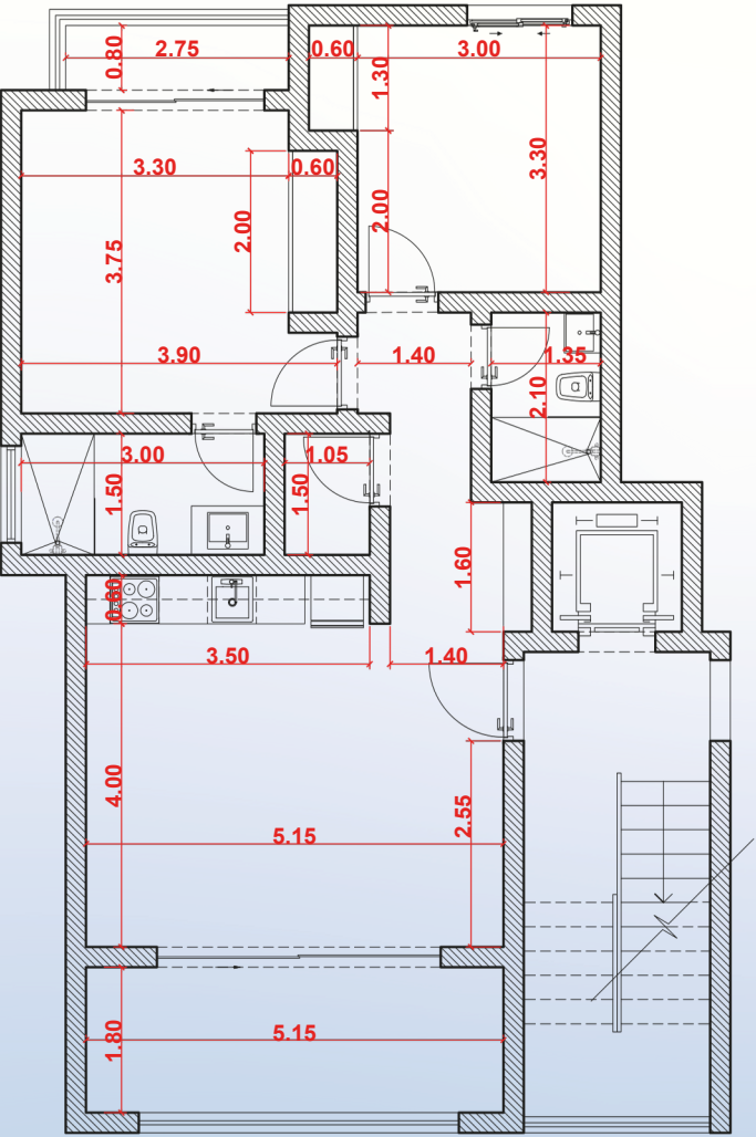
PLANTA DIMENSIONADA
