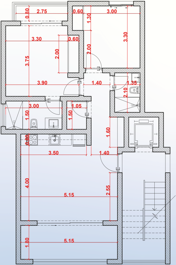
PLANTA DIMENSIONADA
